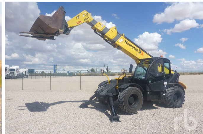
HAULOTTE HTL4017 4X4X4
